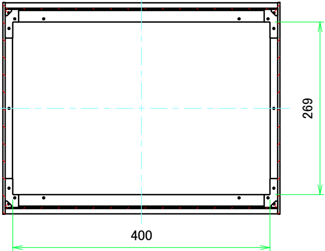
B-B ( 1 : 6 )
