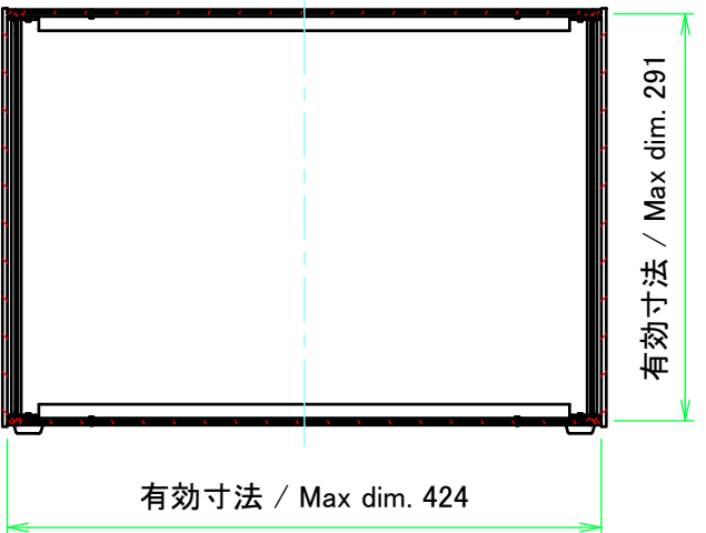
C-C ( 1 : 6 )
